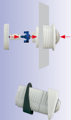
Montage ohne und mit 15°-Keil (Zubehör)
